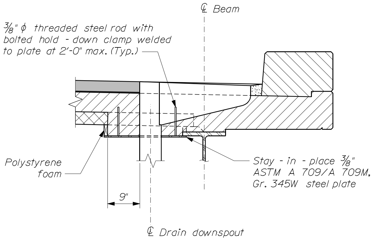
~ SECTION D-D ~
