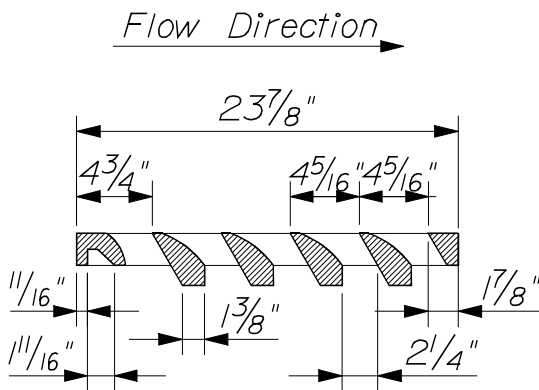
~ SECTION E-E ~
